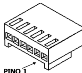
Pinagem do conector CN3
